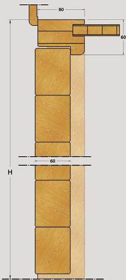
PORTAFINESTRA VISTA INTERNA doghe verticali
